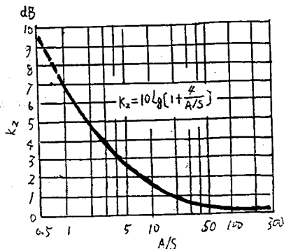
图 A1 环境修正值 K_2 (dB)
