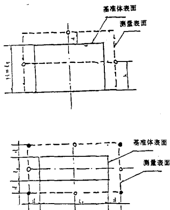
图 1 矩形六面体测量表面上的测点位置
